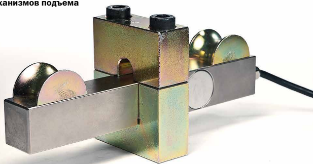
Датчик нагрузки – проверенное в эксплуатации решение для любых механизмов подъема
