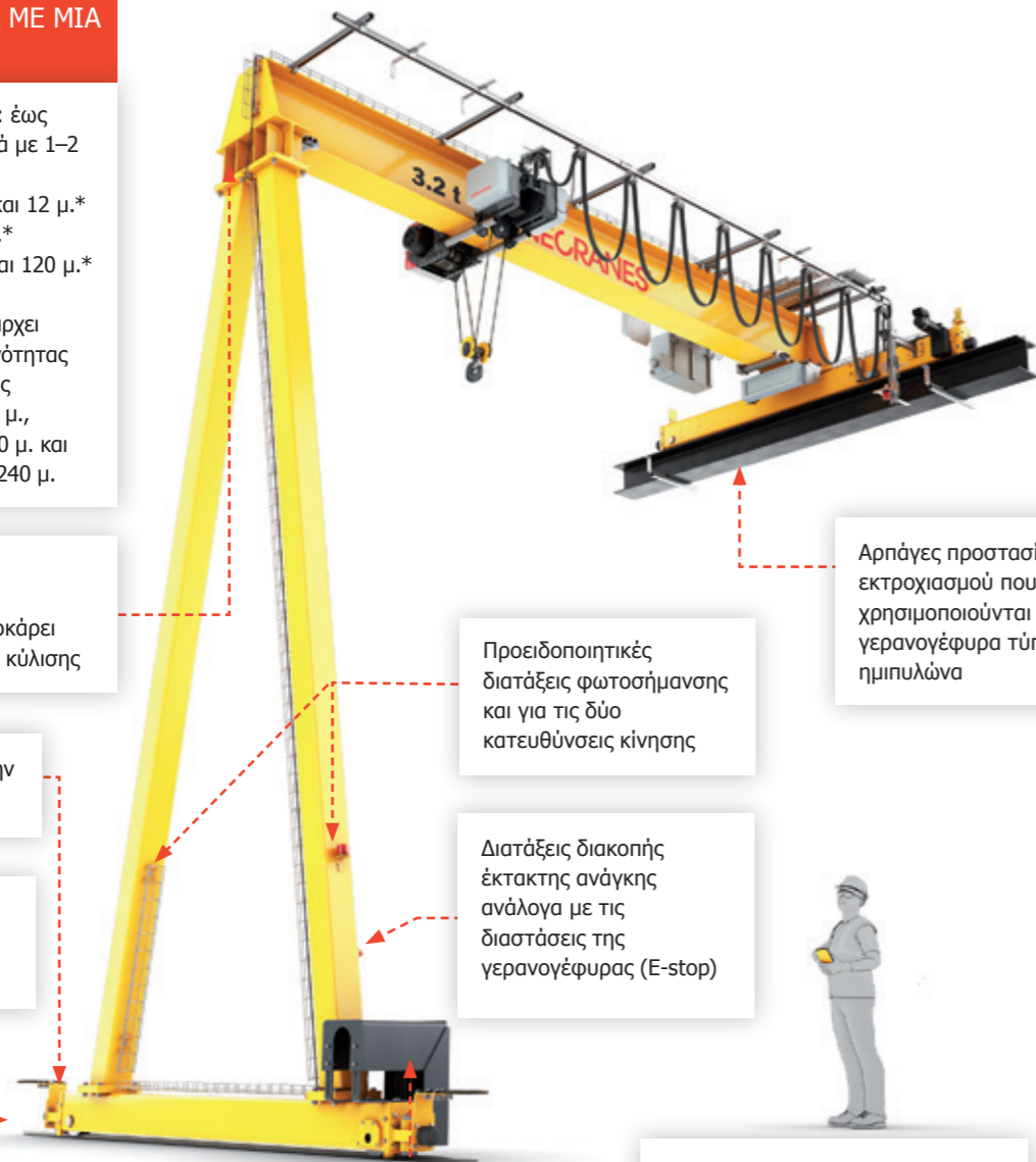
Γερανογέφυρα μονού φορέα ημιπυλώνα
