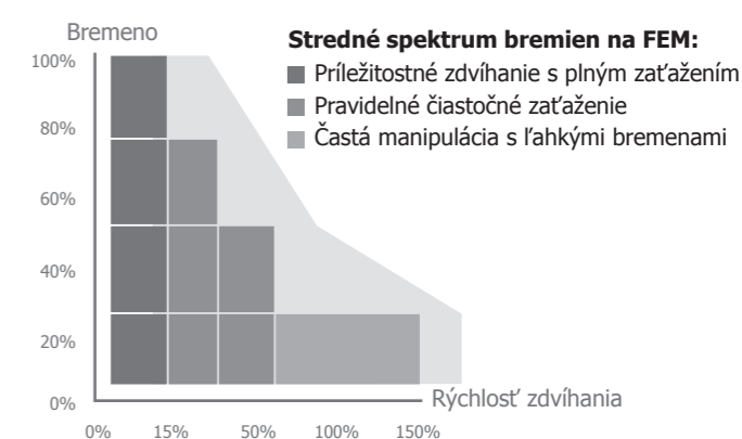
Charakteristika motora pre invertorový kladkostroj (ASR): Vysoká rýchlosť pre ľahké bremená Stredná rýchlosť pre stredne veľké zaťaženie Bezpečná rýchlosť pre ťažké bremená
