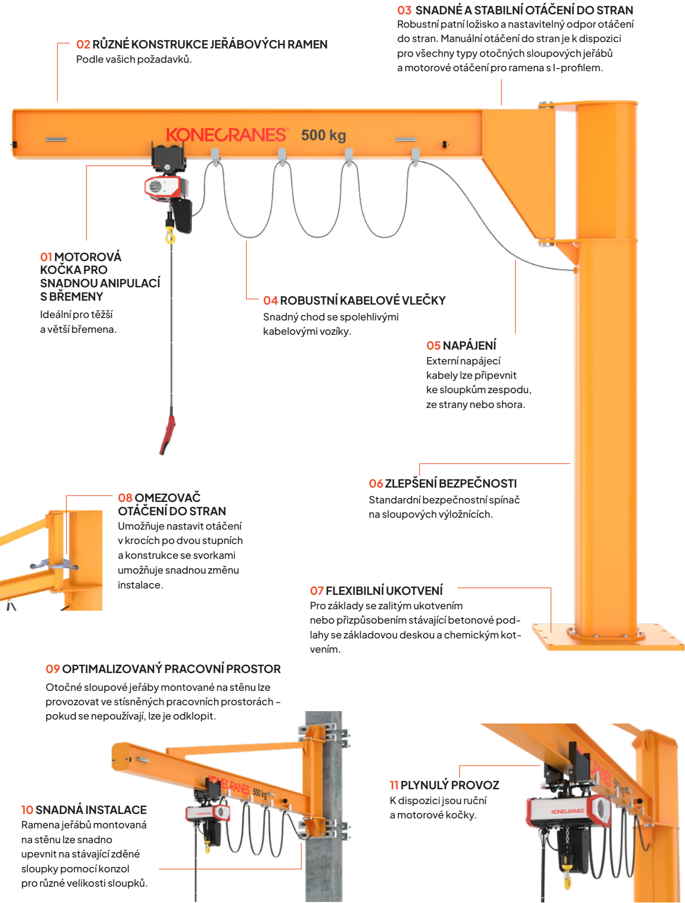
SLOUPOVÝ OTOČNÝ JEŘÁB
